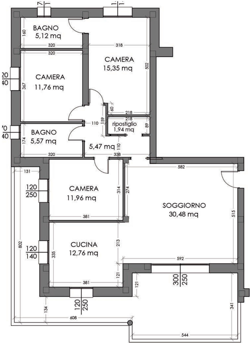
PIANTA QUOTATA
