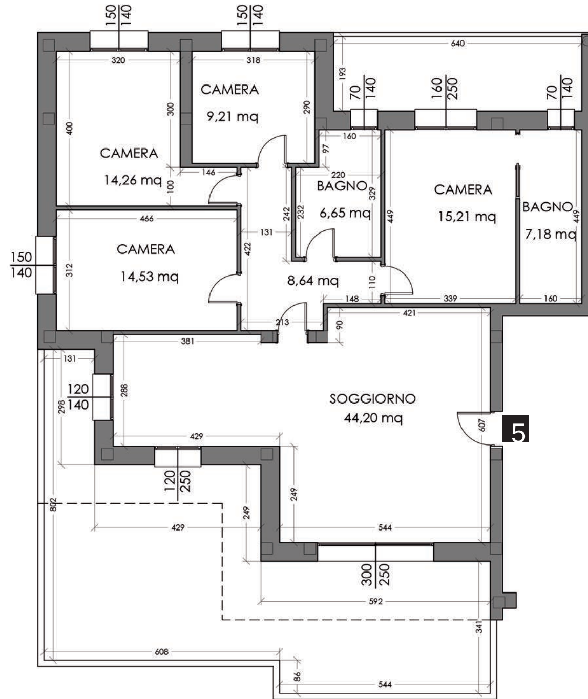
PIANTA QUOTATA
